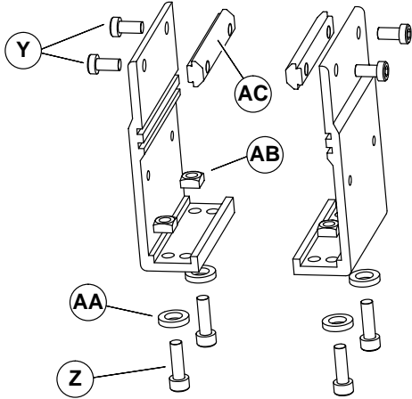
Installationsträger für Flachbandförderer Abbildung 9
