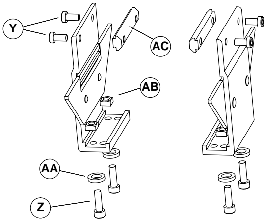
Installationsträger für Stollenförderband Abbildung 10
