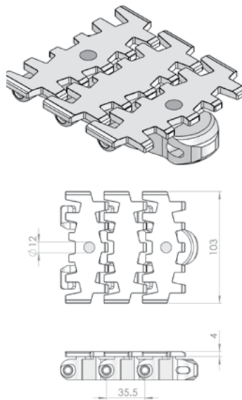
Magnet Top Chain FMMT-5-L#
